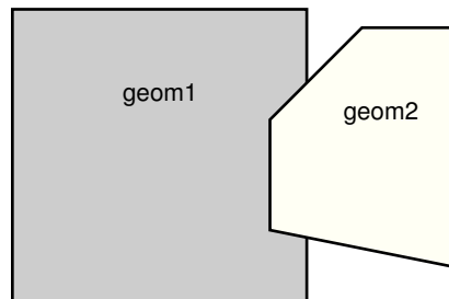
Figure 26-2 SDO_GEOM.SDO_DIFFERENCE
